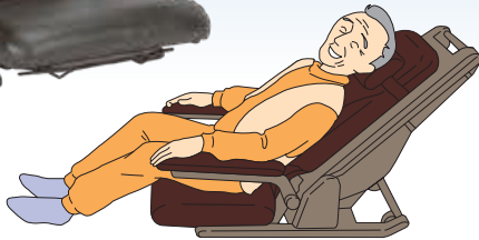
電動チルト機構 背もたれと座板が一緒に傾斜。
